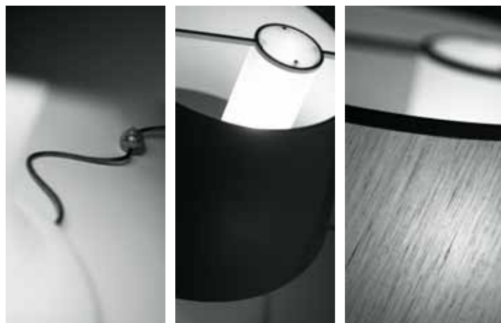
Switch on the cable / Interruptor en el cable. Borosilicate inner glass / Vidrio interior de borosilicato. Lamé diffuser / Tejido especial Lamé.
