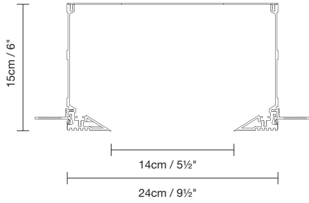
sección caja Deep System
