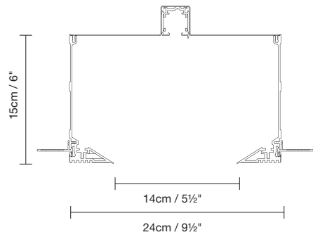
sección caja Deep Track System
